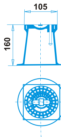
Skrzynka do nawierarki - niska Box for spotting drill Ящик к засверловке
