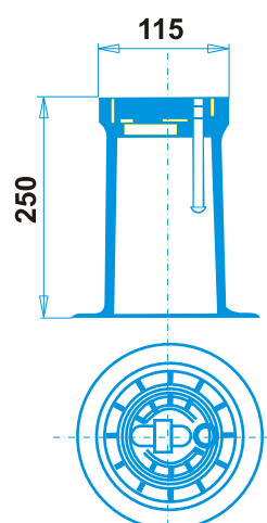
Skrzynka do nawierarki - wysoka Box for spotting drill road Ящик к уличной засверловке
